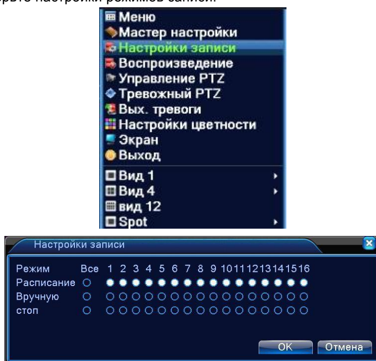
Рисунок 3.7 Режимы записи
