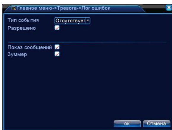
Рисунок 4.11 Лог ошибок
