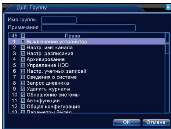
Рисунок 4.48 Добавить группу
