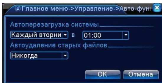
Рисунок 4.51 Автоматическое обслуживание
