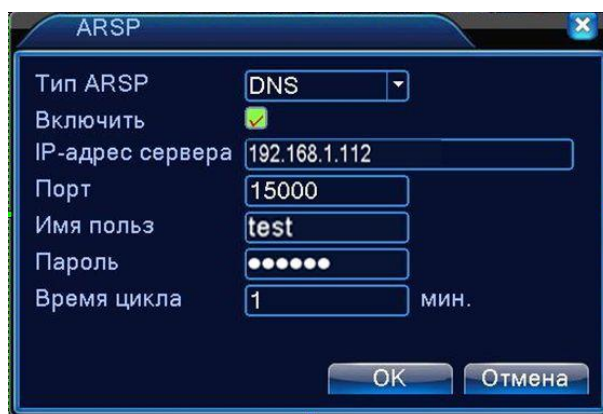
Рисунок 4.29 ARSP
