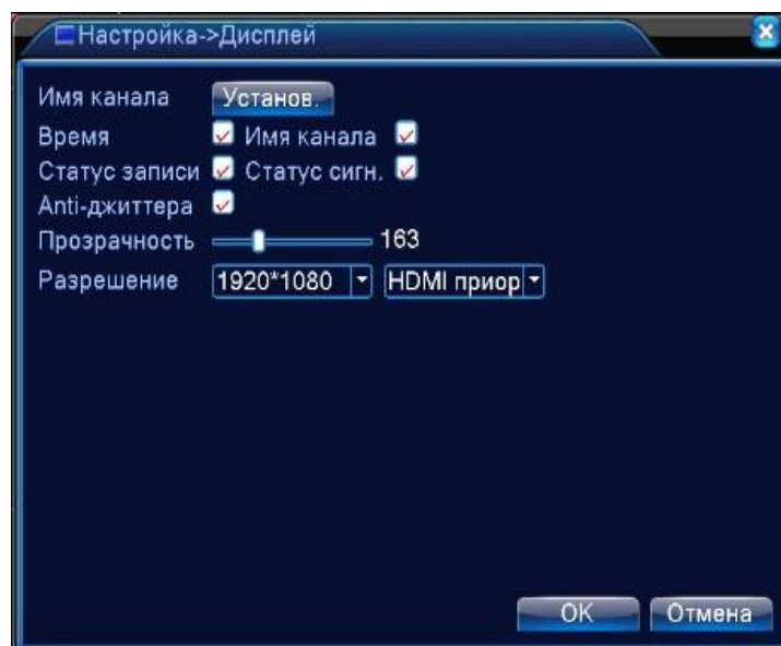
Рисунок 4.36 Отображение
