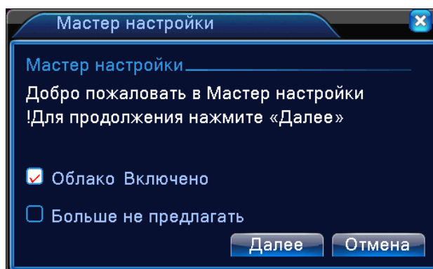
Рисунок 3.3 Режим «Облако».
