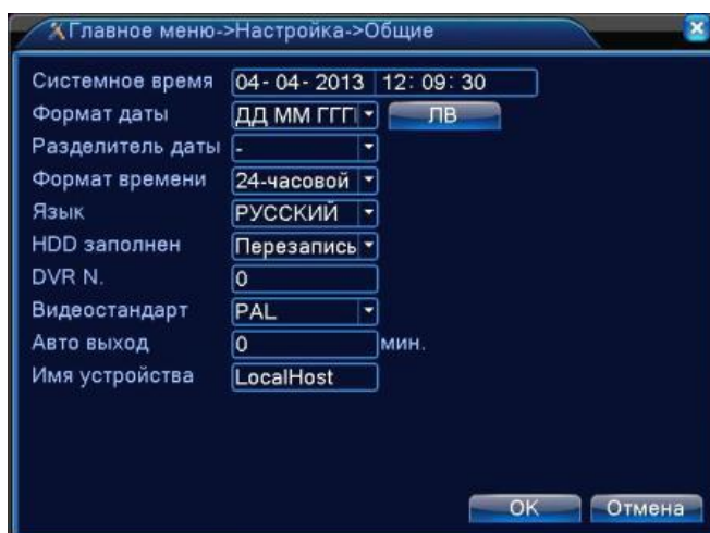
Рисунок 4.17 Общие настройки
